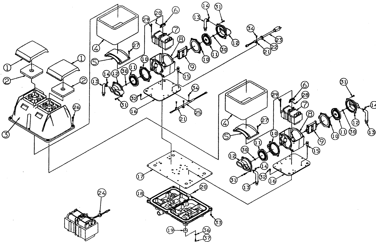
ソレノイド部組立図
